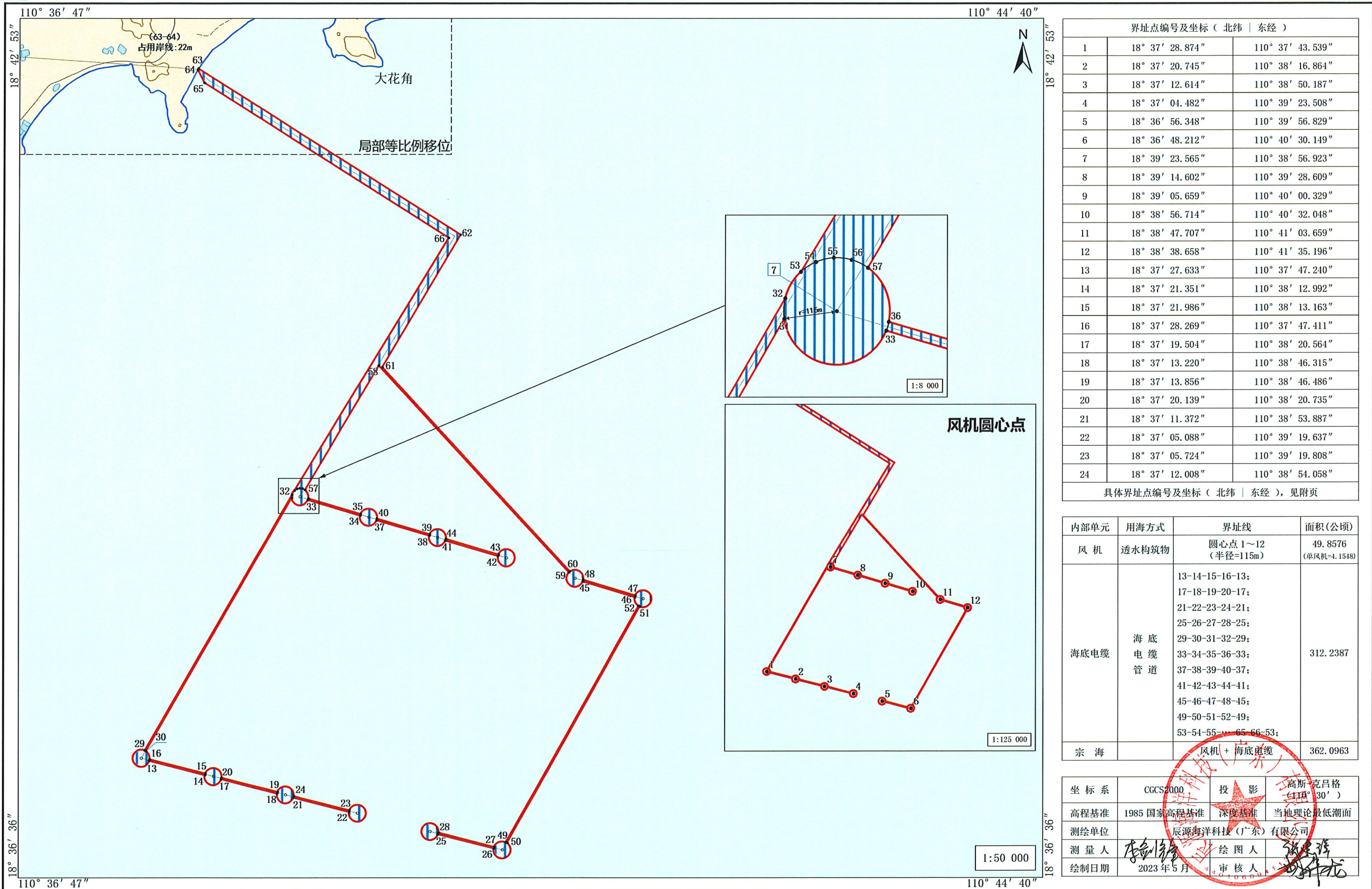
中电建万宁漂浮式海上风电试验项目一期工程宗海界址图
