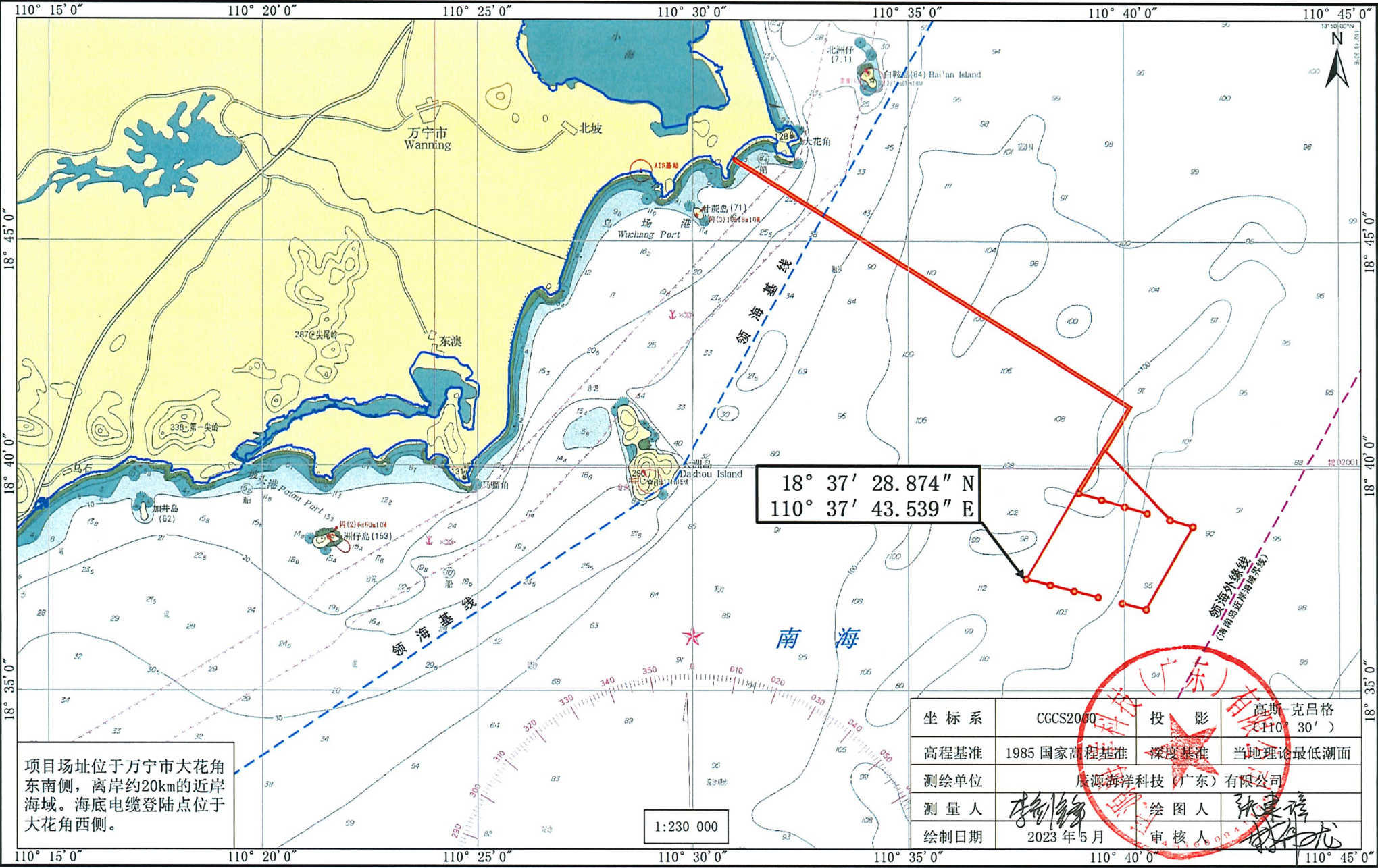
中电建万宁漂浮式海上风电试验项目一期工程宗海位置图
