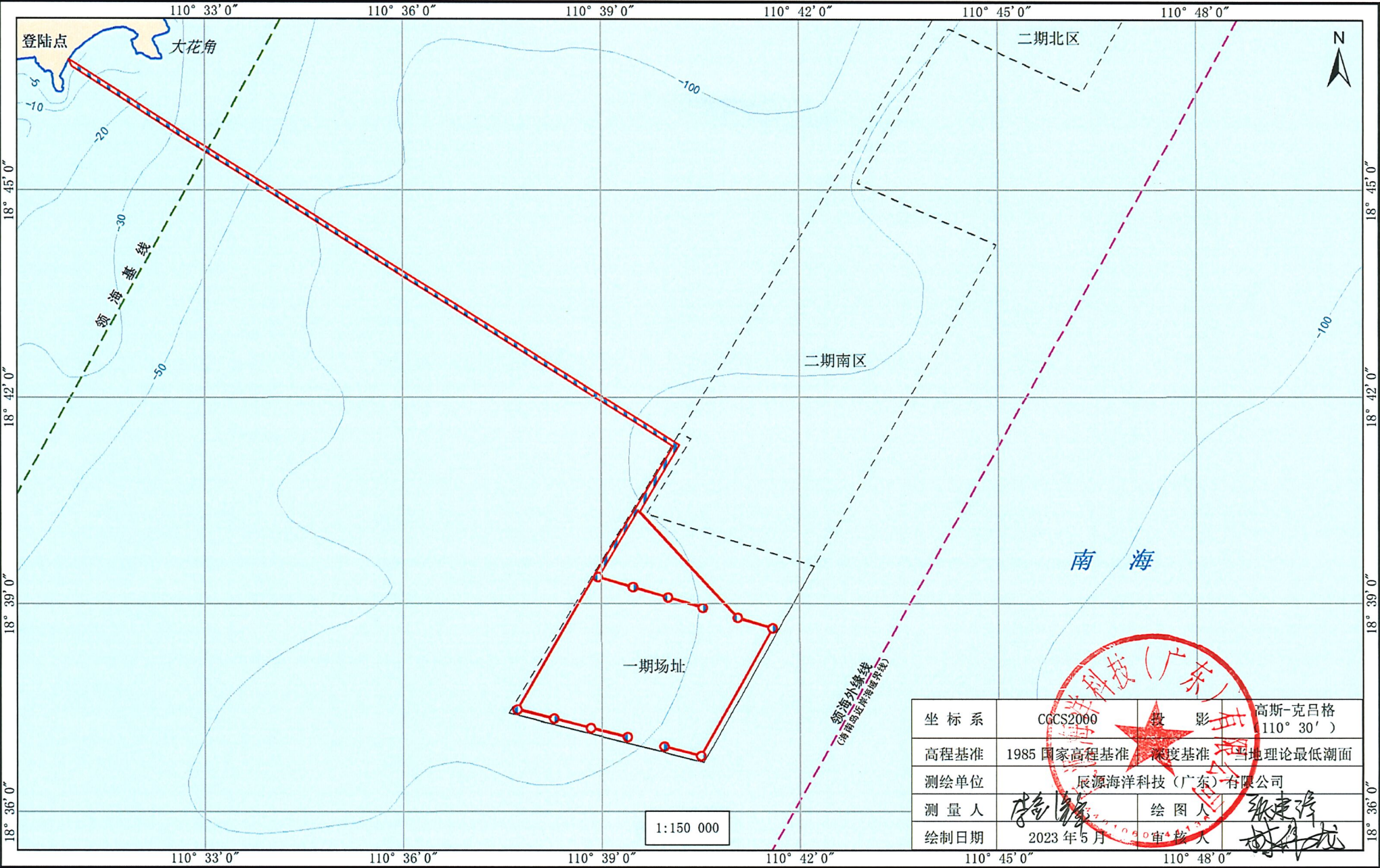
中电建万宁漂浮式海上风电试验项目一期工程宗海平面布置图
